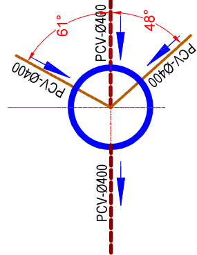
Podłączenia studni S-3
