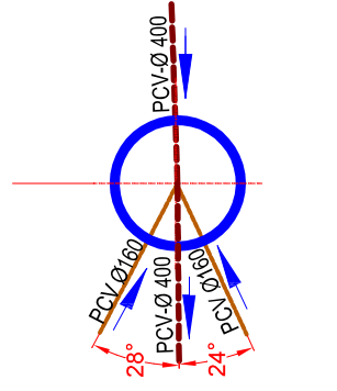
Podłączenia studni S-1
