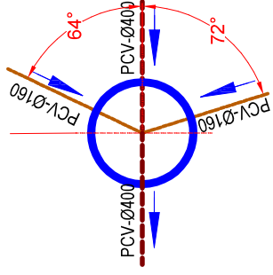
Podłączenia studni S-2
