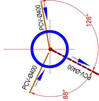
Podłączenia studni S-5
