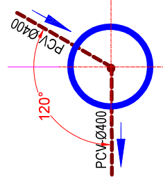
Podłączenia studni S-4
