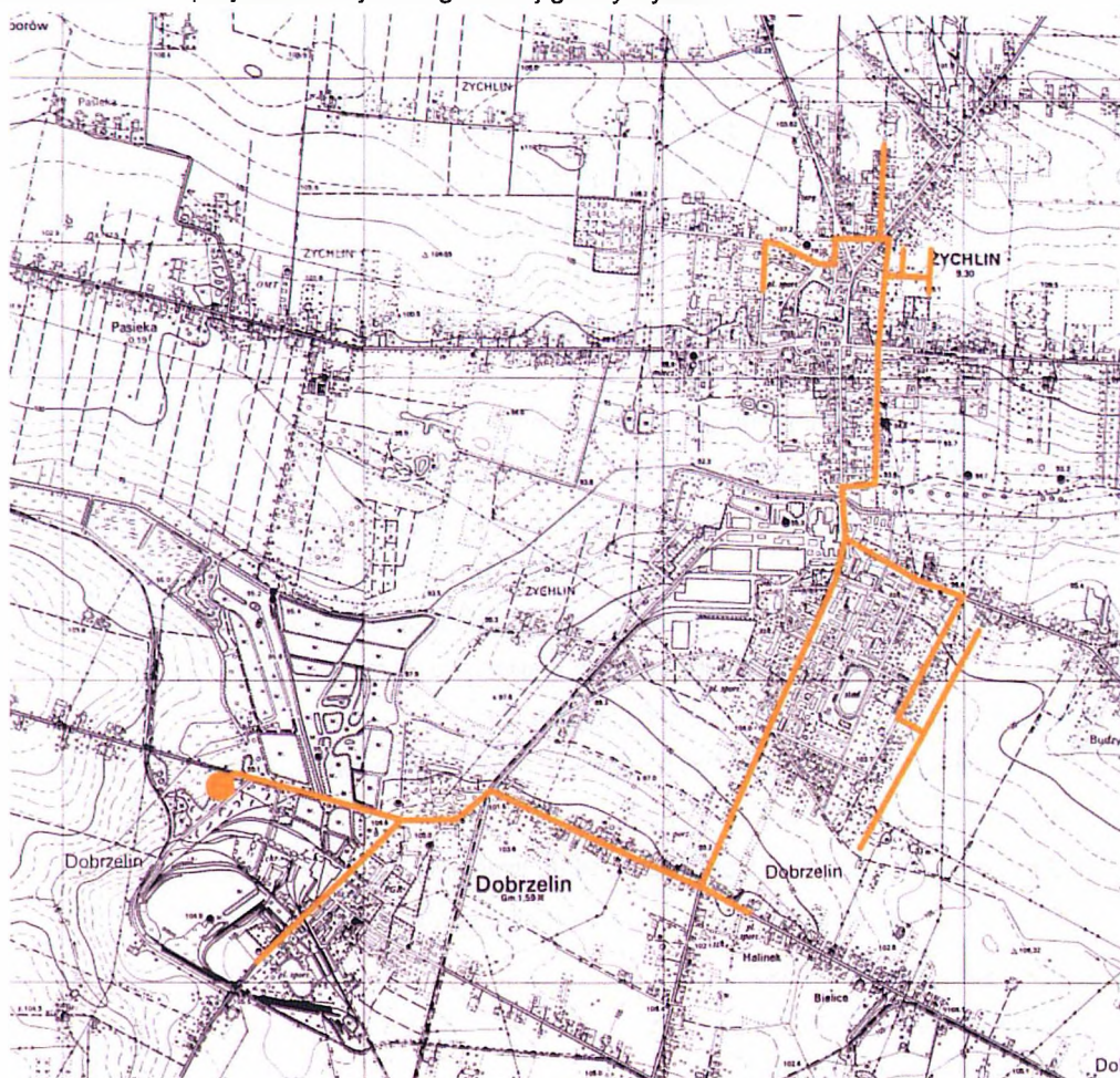
Rysunek 5 Schemat projektowanej sieci gazowej gminy Żychlin
