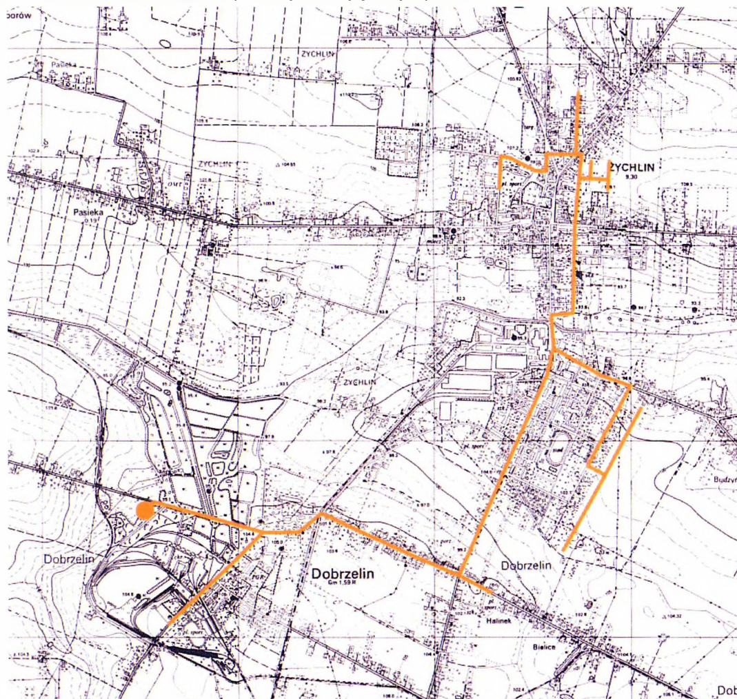
Rysunek 5 Schemat projektowanej sieci gazowej gminy Żychlin
